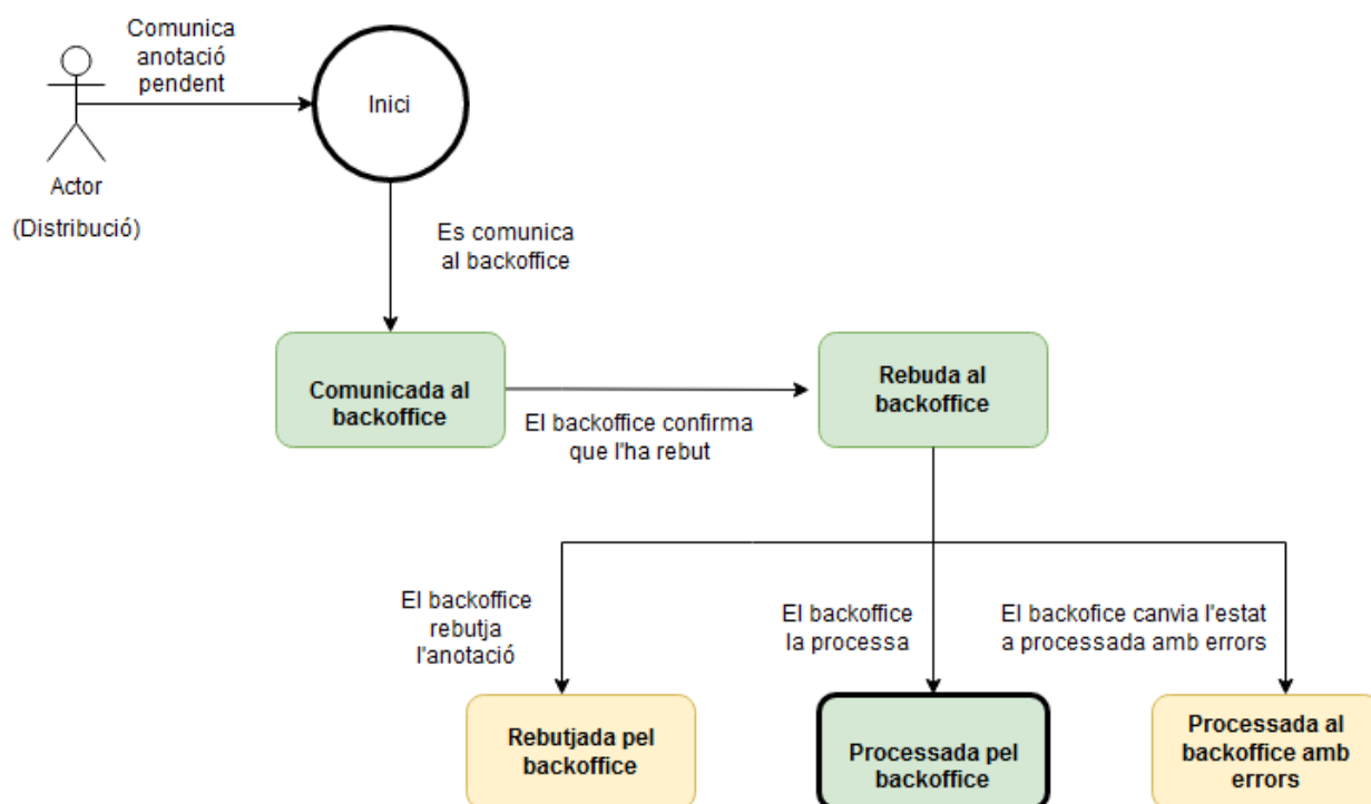
fig. 15: Diagrama d'estat: procés d'una anotació quan es comunica amb el backoffice
