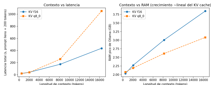
Figure 5: Contexto vs latencia y RAM
