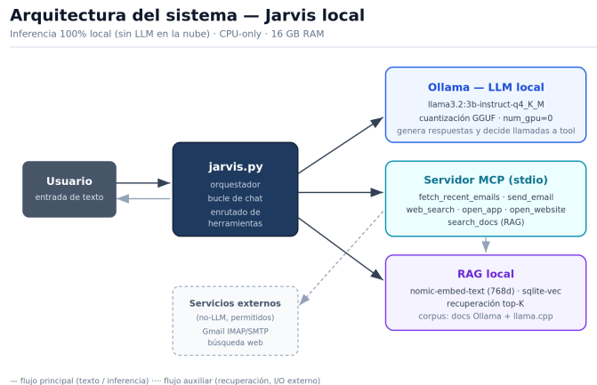
Figure 1: Arquitectura del sistema
