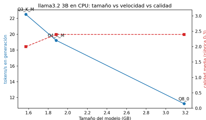
Figure 4: Tamaño vs velocidad vs calidad
