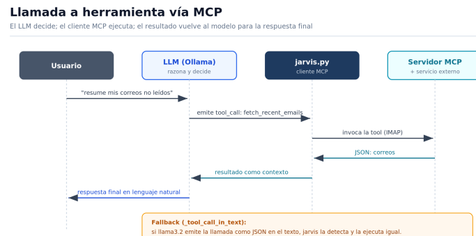
Figure 3: Llamada a herramienta vía MCP
