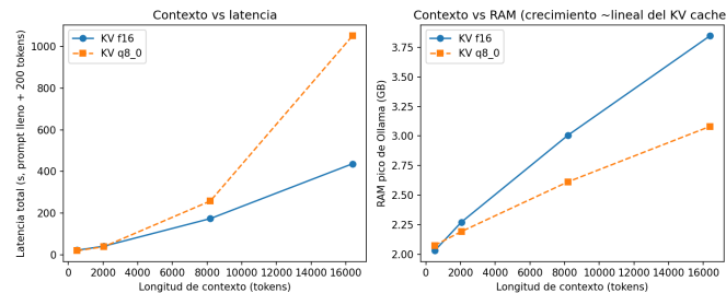
Figure 5: Contexto vs latencia y RAM
