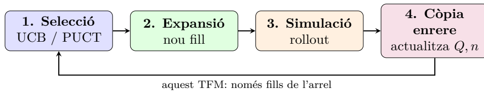
Figura 2.5: Cicle clàssic de l'MCTS adaptat a simulacions de 5 torns a l'arrel.
