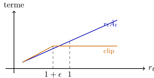
Figura 2.6: Intuïció de l'objectiu retallat de PPO.
