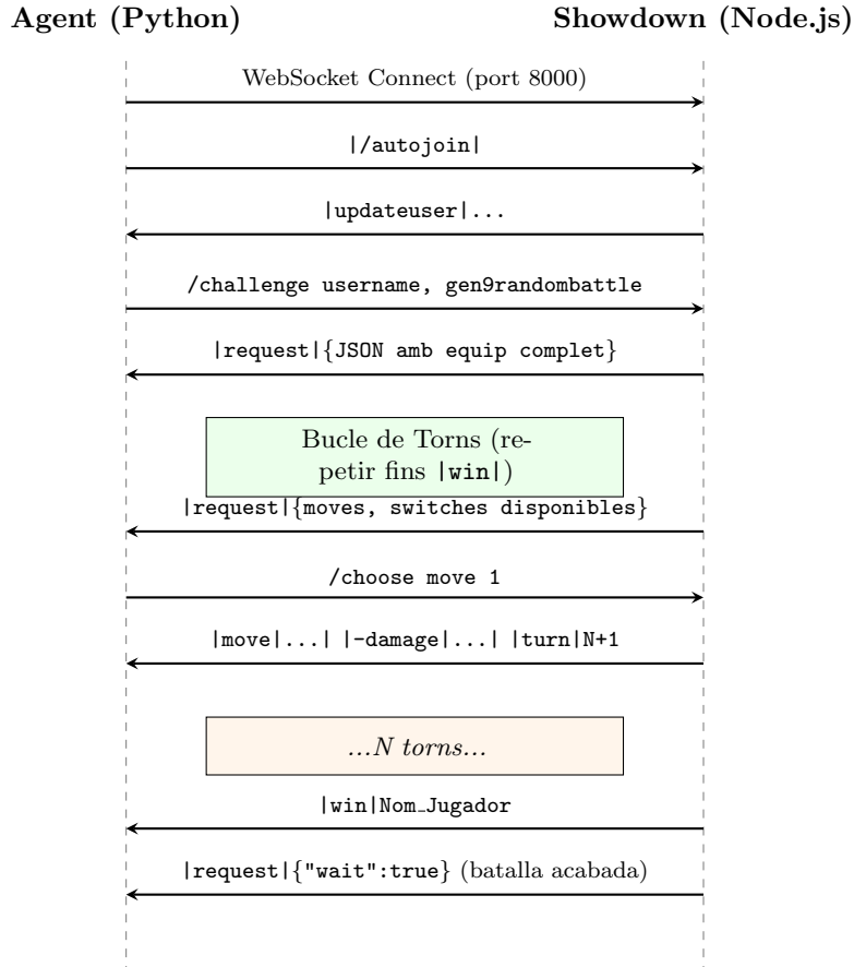
Figura 3.1: Diagrama de seqüència del protocol WebSocket entre un agent i Pokémon Showdown durant una batalla completa.
