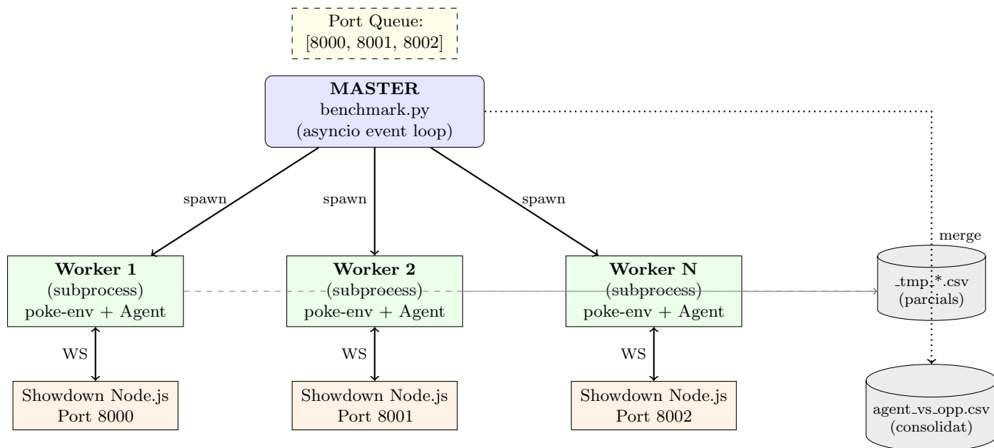
Figura 5.1: Arquitectura completa del sistema Master-Worker. Les línies contínues representen comunicació en RAM (processos i WebSocket), les discontinues representen escriptures a disc (persistència).
