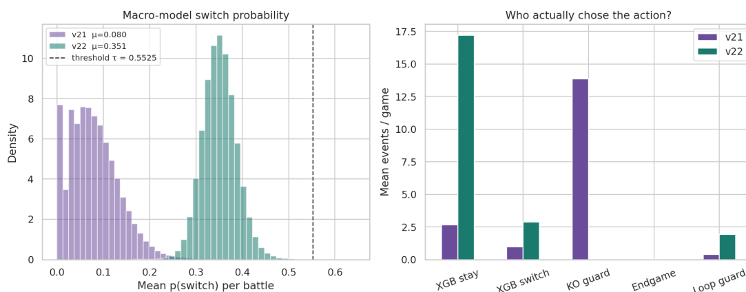
Figura 6.27: Frequència d'ús de la política apresada. XGBoost intervé en el 15% dels torns de v21 i en el 80% dels de v22.
