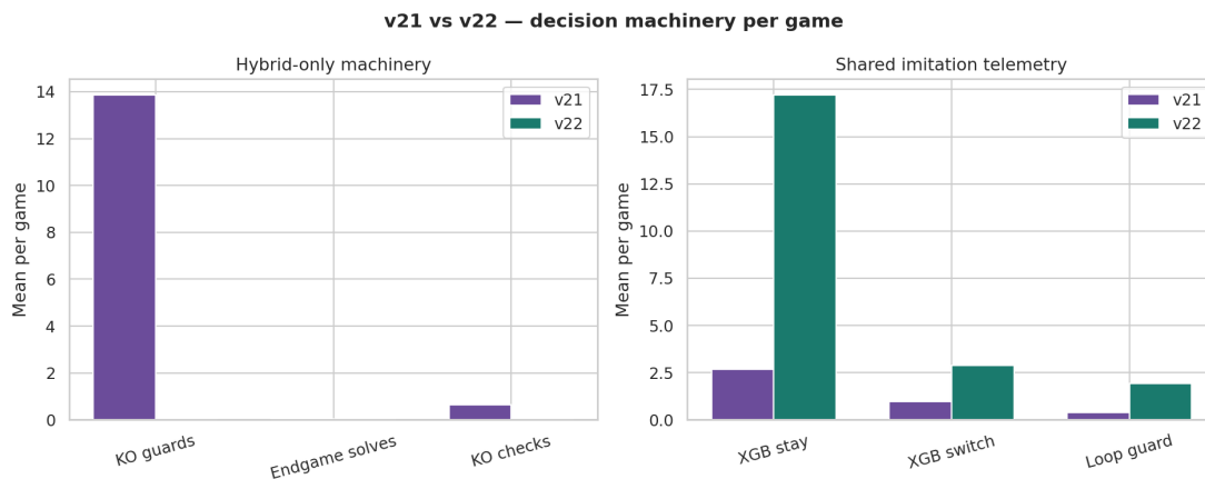
Figura 6.26: Empremta dels agents d'imitació. v21 registra aproximadament 14 proteccions de debilitament per partida i consulta XGBoost en el 15% dels torns. v22 no té aquestes proteccions, consulta XGBoost en el 80% dels torns i activa la protecció de bucle en el 97% de les partides.
