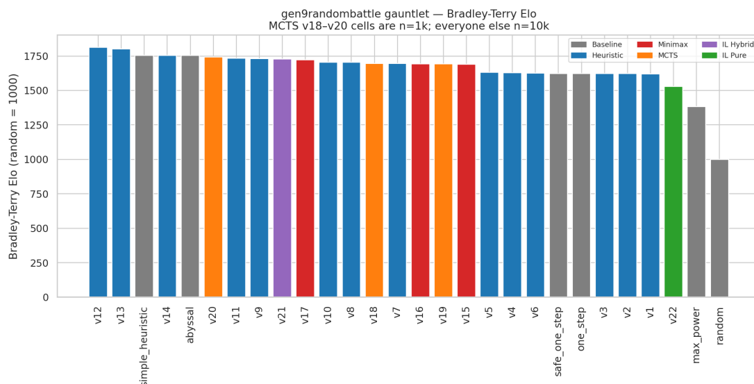
Figura 6.34: Escala latent Bradley-Terry ancorada a random = 1000 ajustada sobre les dues orientacions de la matriu. v12 i v13 obtenen les puntuacions més altes; v14 , Abyssal i Simple Heuristic comparteixen un altiplà a 1755 punts. Les files i columnes d' MCTS aporten una desena part de partides al model ( n = 1.000 ).
