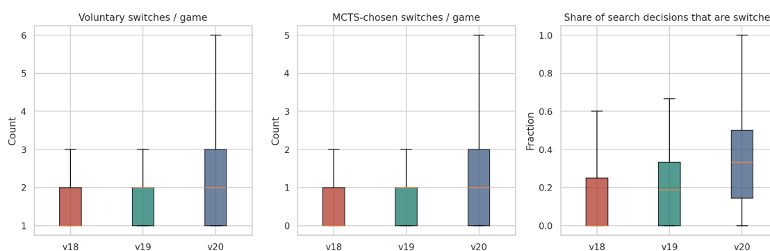
Figura 6.22: Distribució dels canvis a MCTS. PUCT augmenta la fracció de decisions de cerca que acaben en canvi i amplia la distribució de canvis voluntaris.
