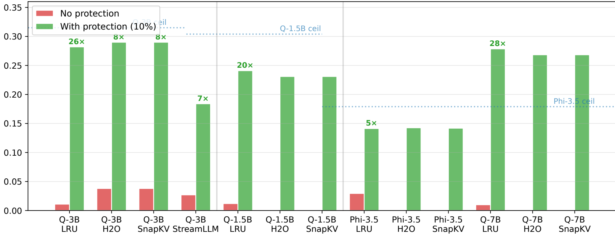
Token F1 (C = 256)
