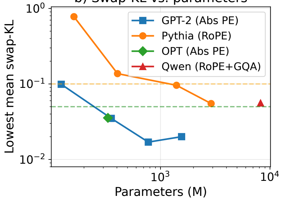
b) Swap-KL vs. parameters
