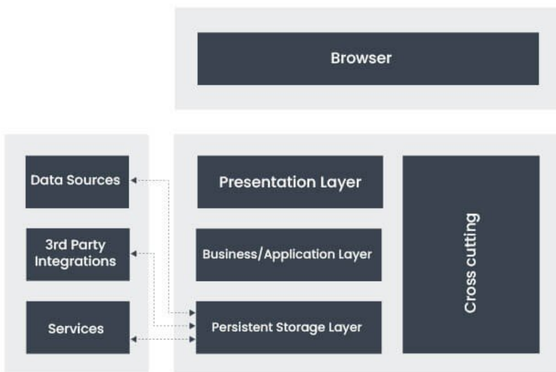
Rys. 8. Diagram, przedstawiający warstwy aplikacji internetowej. Źródło: https://www.albiorixtech.com/wp-content/uploads/2025/12/web-application-architecture-layers.jpg (dostęp: 03.02.2026)
