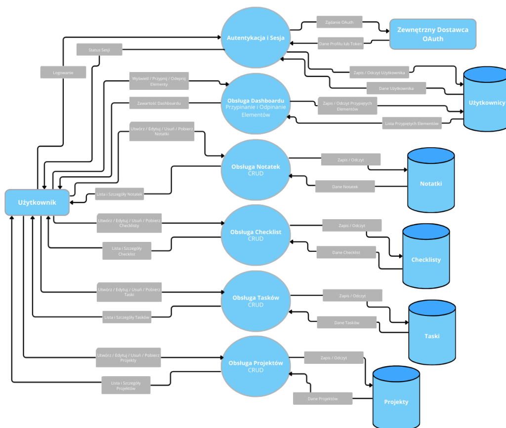
Rys. 11. Diagram przepływu danych poziomy 1
