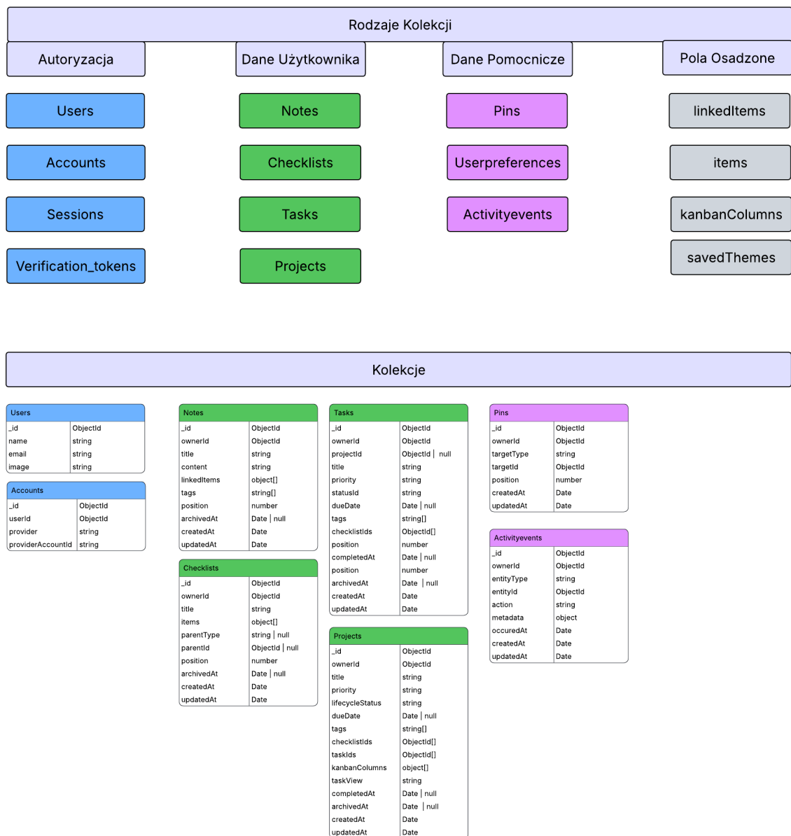
Rys. 13. Schemat struktury bazy danych aplikacji.
