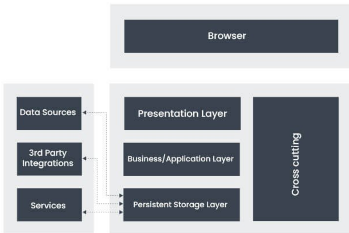
Rys. 9. Diagram, przedstawiający warstwy aplikacji internetowej. Źródło: [1], https://www.albiorixtech.com/wp-content/uploads/2025/12/web-application-architecture-layers.jpg (dostęp: 03.02.2026).
