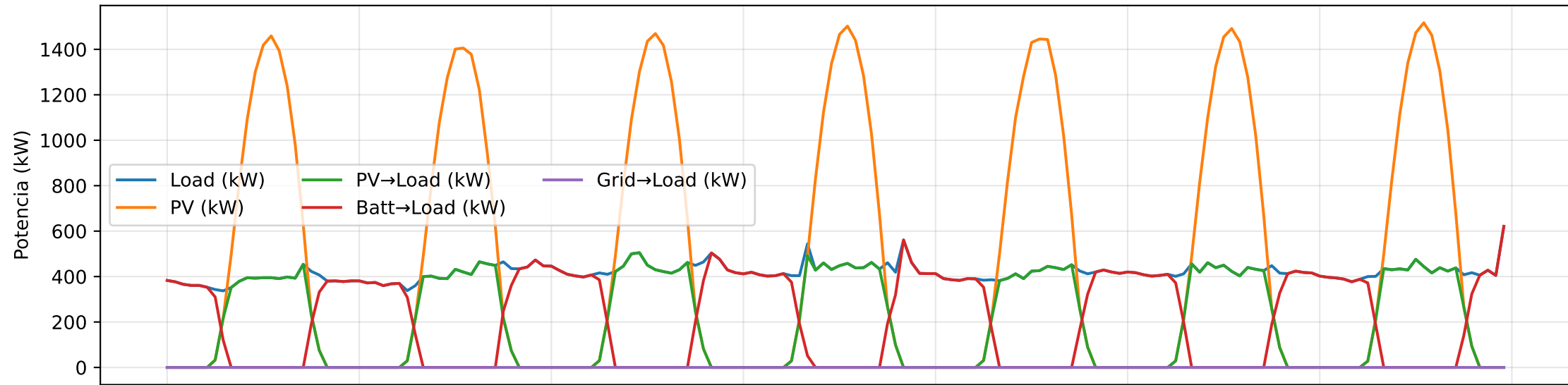
Acoplamiento FV-Carga-Batería (ventana semanal)
