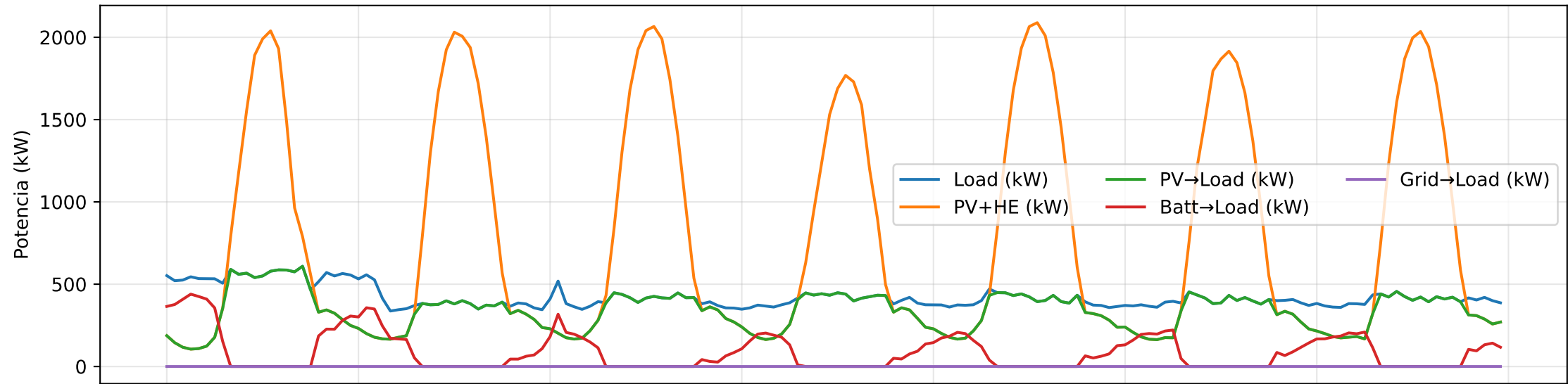
Acoplamiento FV+HE-Carga-Batería (ventana semanal)
