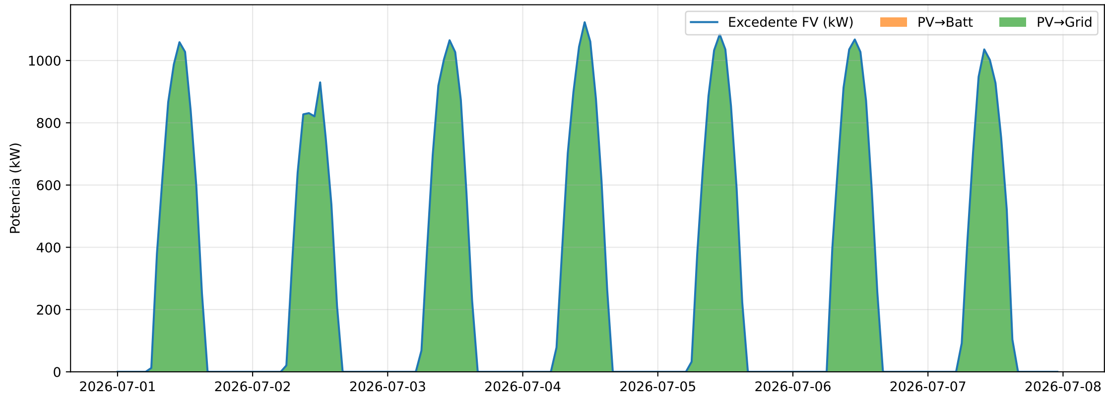
Gestión del excedente fotovoltaico (stack)
