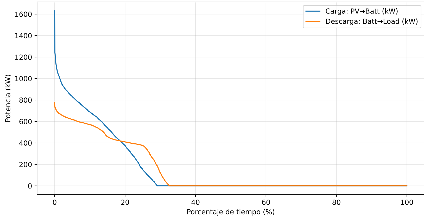
Curvas de duración de potencia (carga/descarga)
