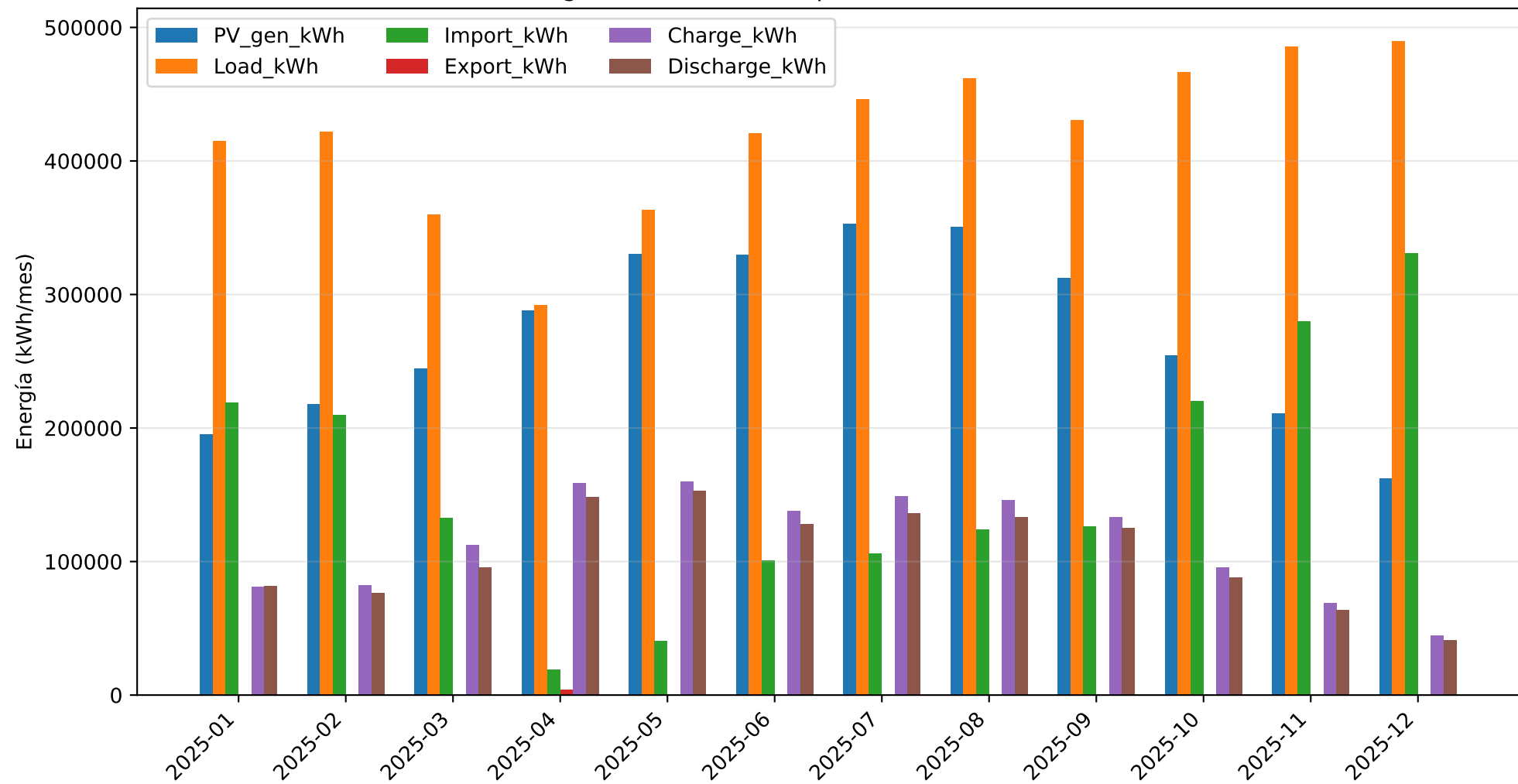
Energías mensuales (acoplamiento FV-Batería-Red)
