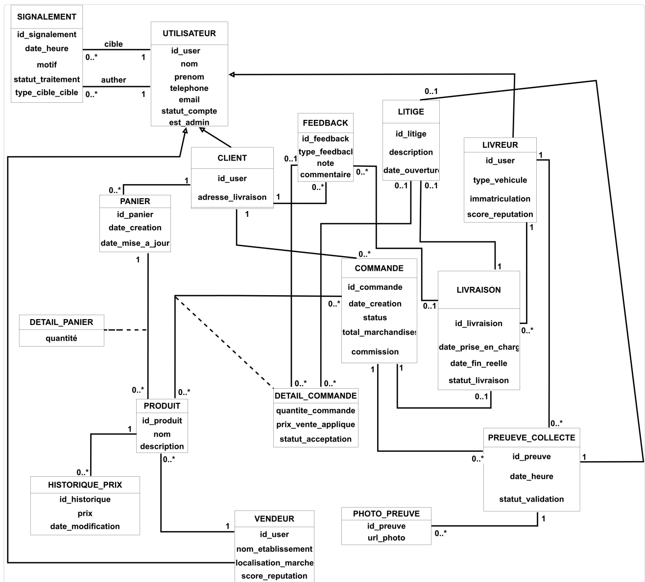
Figure 2 : Diagramme de Classes.
