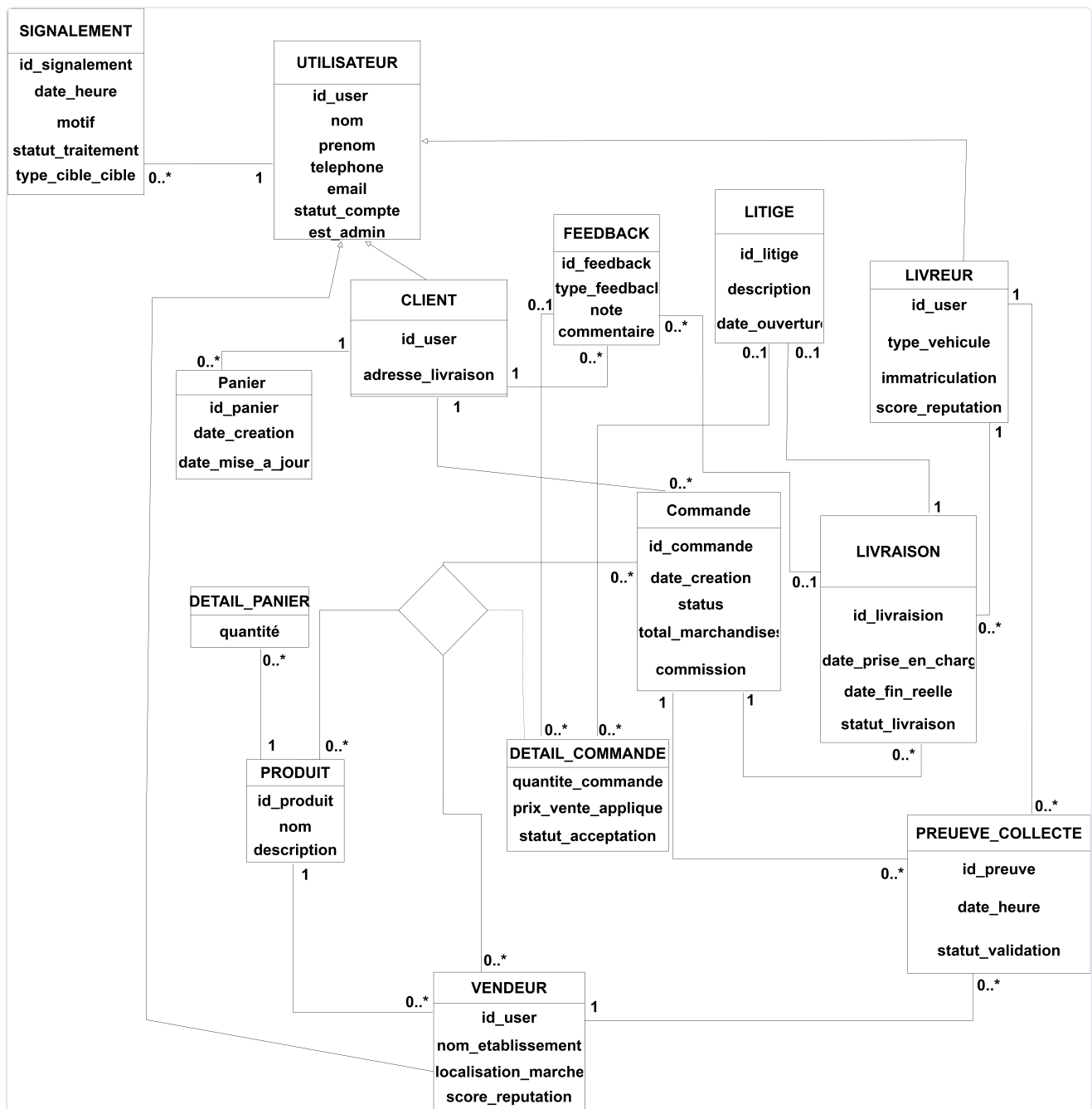
Figure 2 : Diagramme de Classes.
