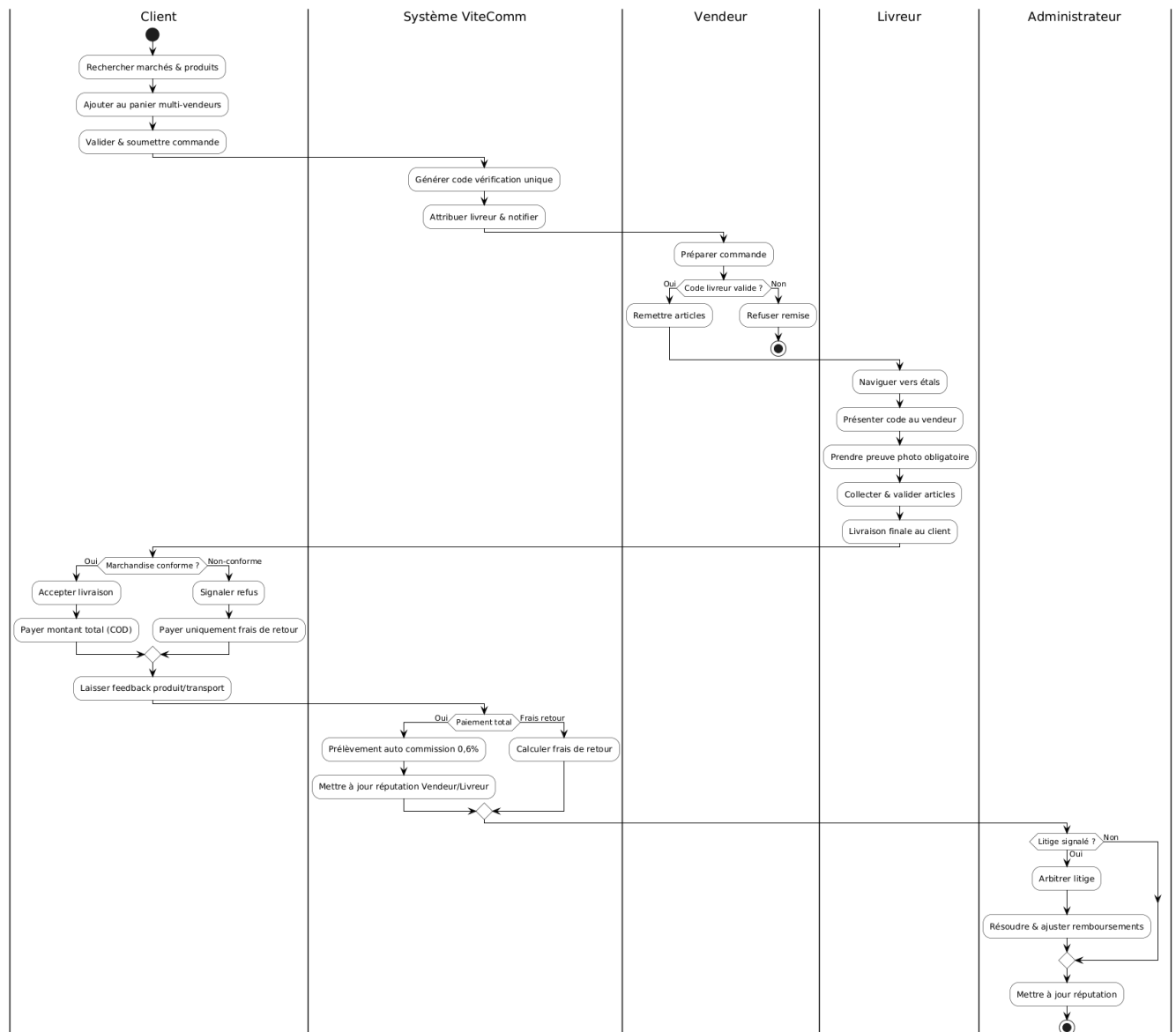
Figure 3 : Diagramme d'Activité.
