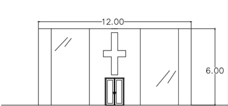
FACHADA FRONTAL
