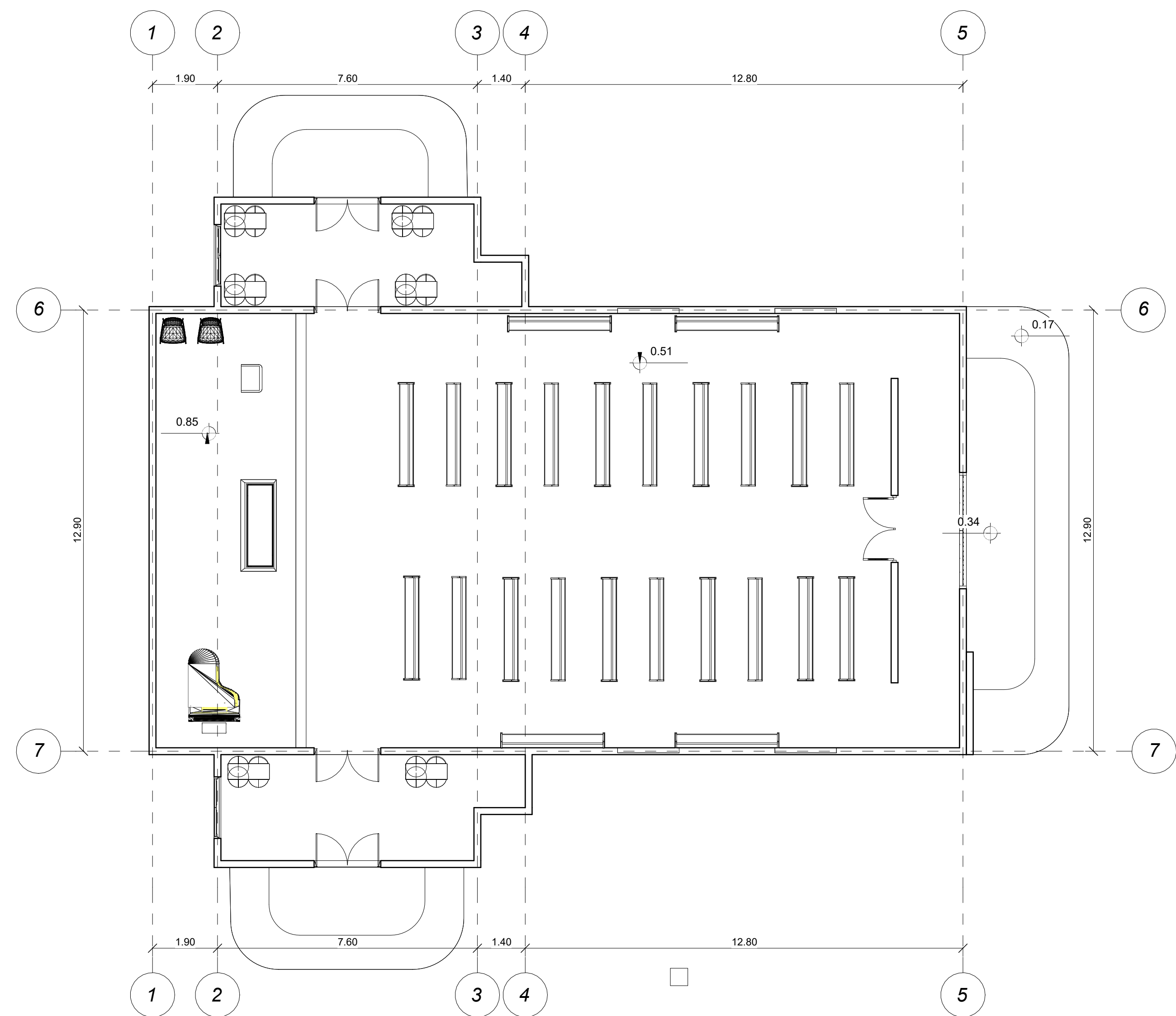
PLANTA ARQUITECTONICA BAJA
