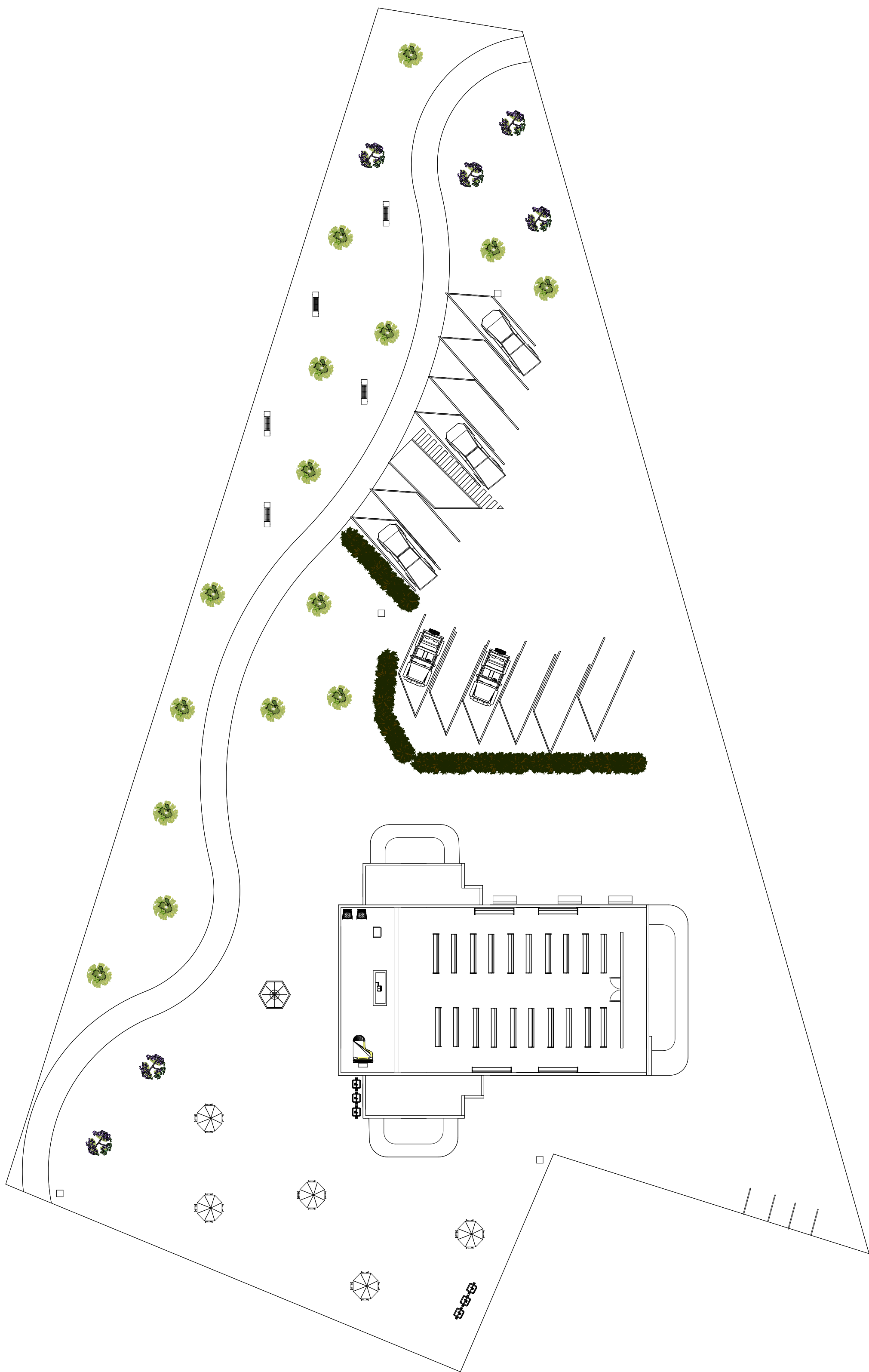
PLANTA ARQUITECTONICA DE CONJUNTO
