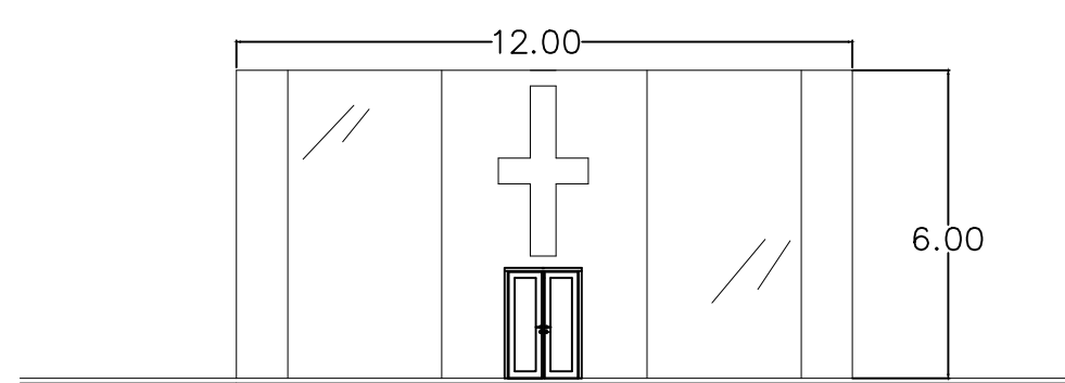
FACHADA FRONTAL
