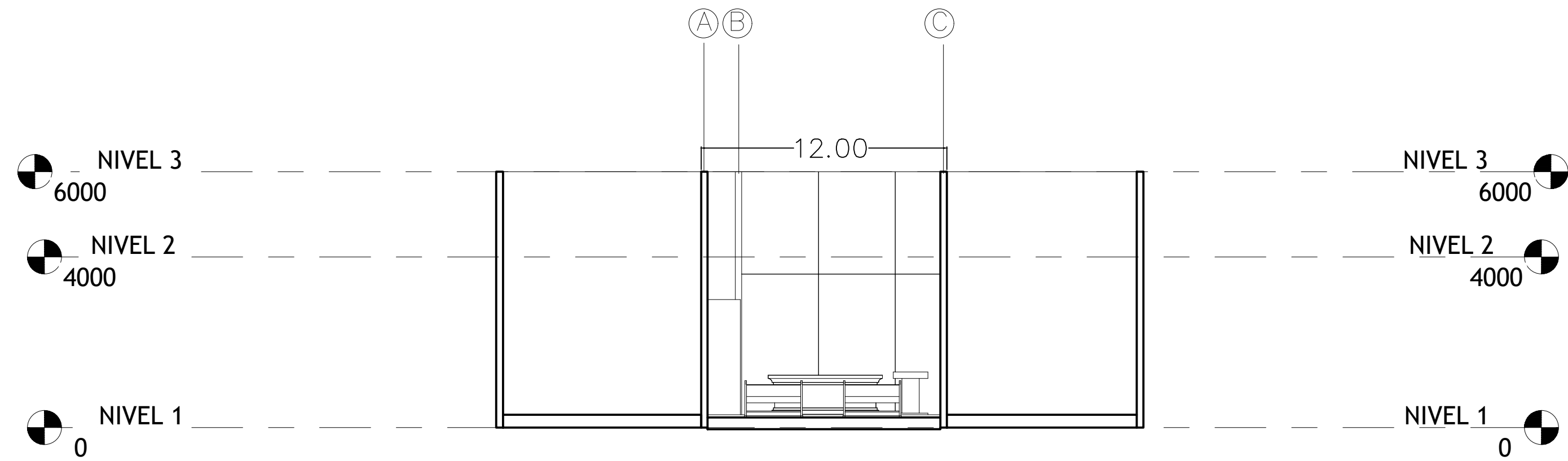
CORTE TRANSVERSAL
