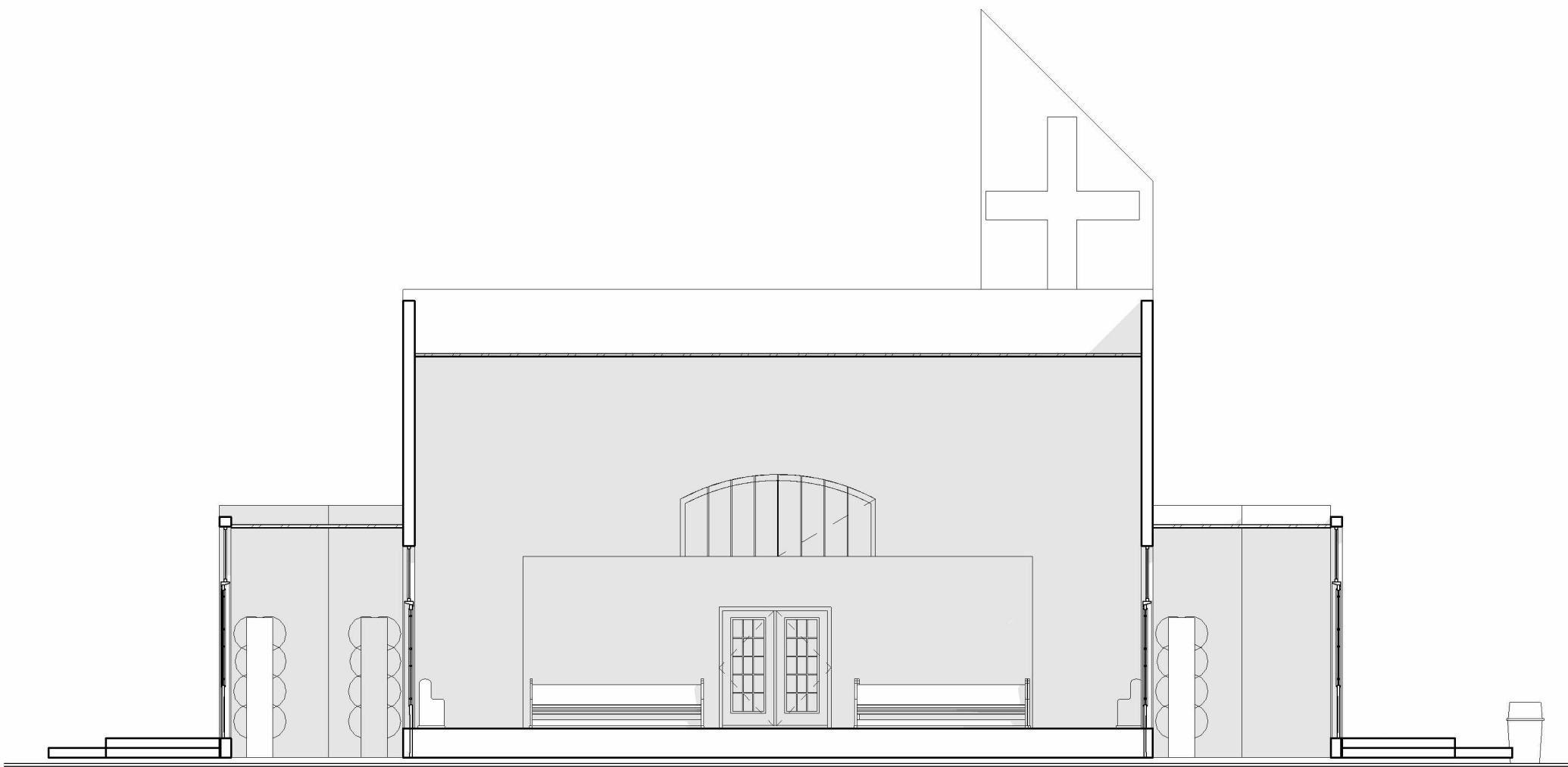
CORTE TRANSVERSAL
