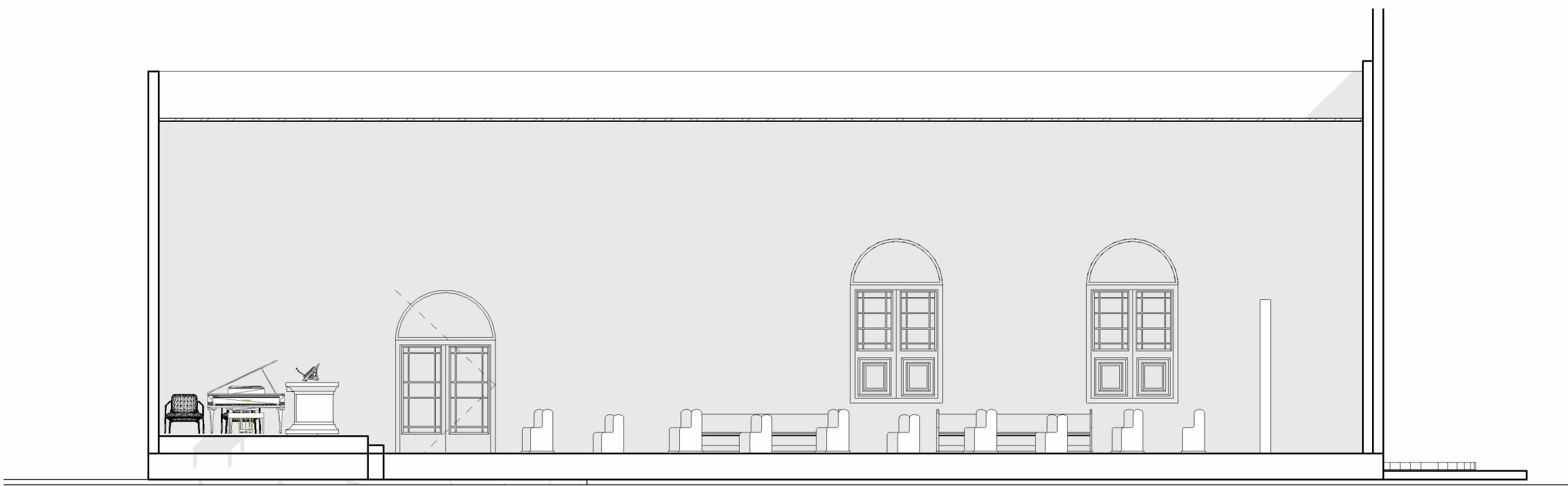
CORTE LONGITUDINAL
