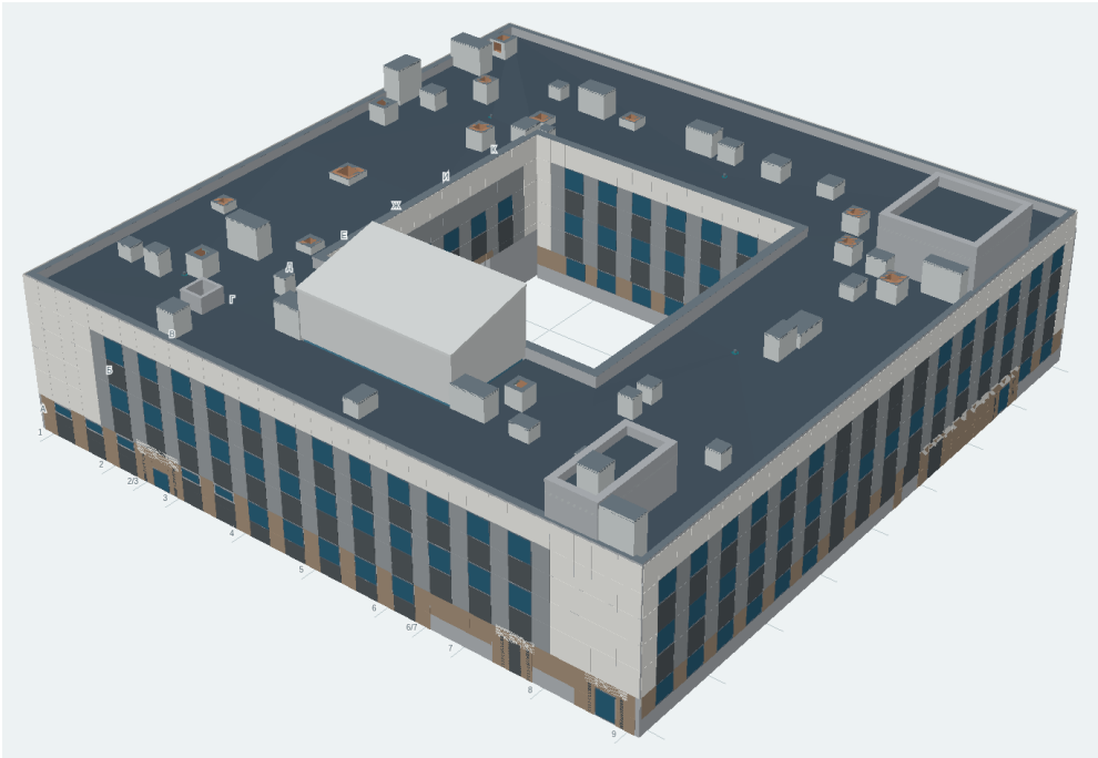
Общий вид R02. Изображение получено из редактируемой модели; не генеративная визуализация.
