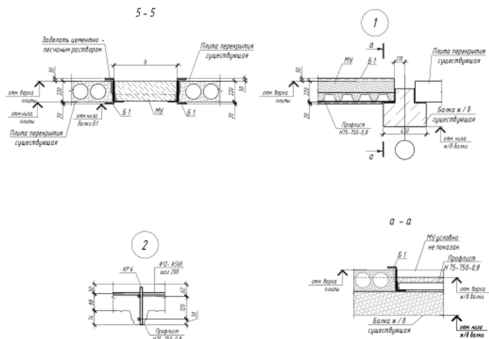
Фрагмент исходного л.24 (PDF 25): опирание Б1 на существующий ригель, сечение и профлист. В чертеже встречаются 110/125 мм; обмерная геометрия ригелей и монтажная увязка не подтверждены.
