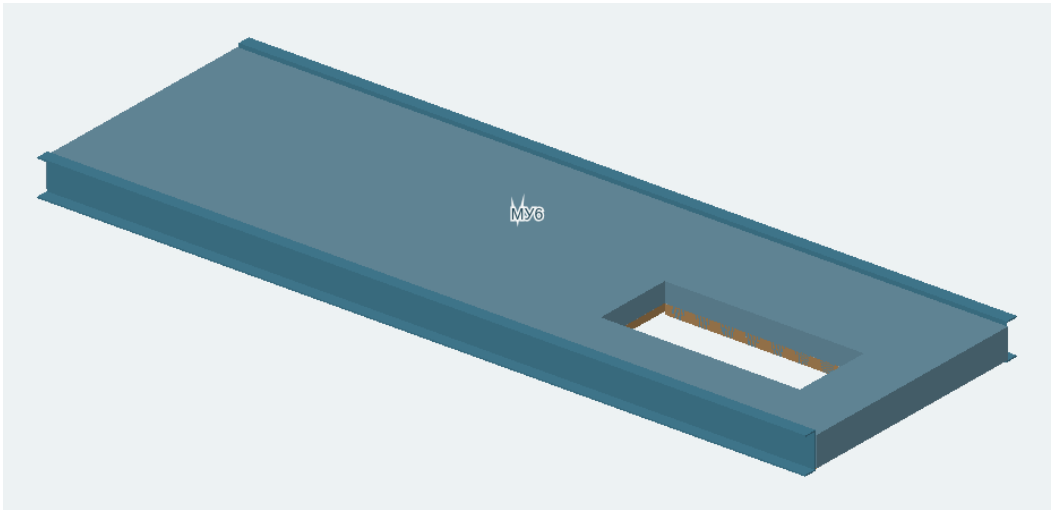
МУ6 в модели: геометрия балки, профлиста, бетона и отверстия. Для просмотра снизу модель можно вращать; общий режим «Усиление · только металл» отключает бетон.
