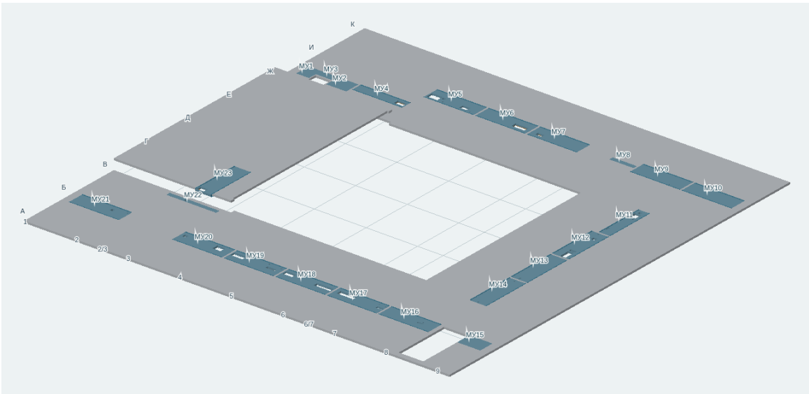
Перекрытие над первым этажом: МУ выделены. Серый контекст — оболочка существующего перекрытия, а не индивидуальная раскладка пустотных плит.
