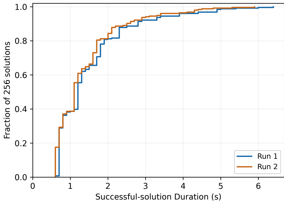
EvolveGPU
