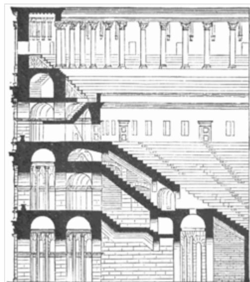
Sezione del Colosseo
