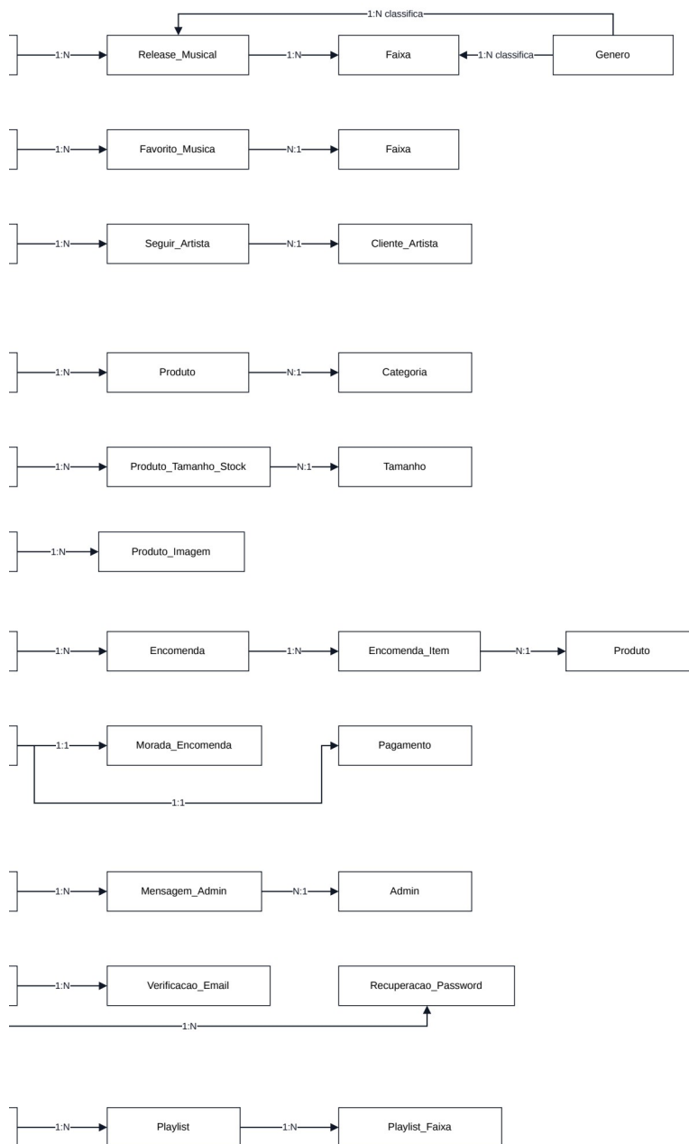
Figura 3.1 - MER compacto, parte 1.
