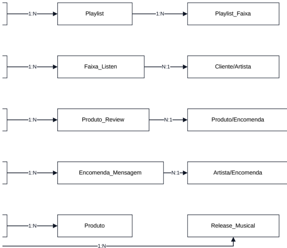
Figura 3.2 - MER compacto, parte 2.
