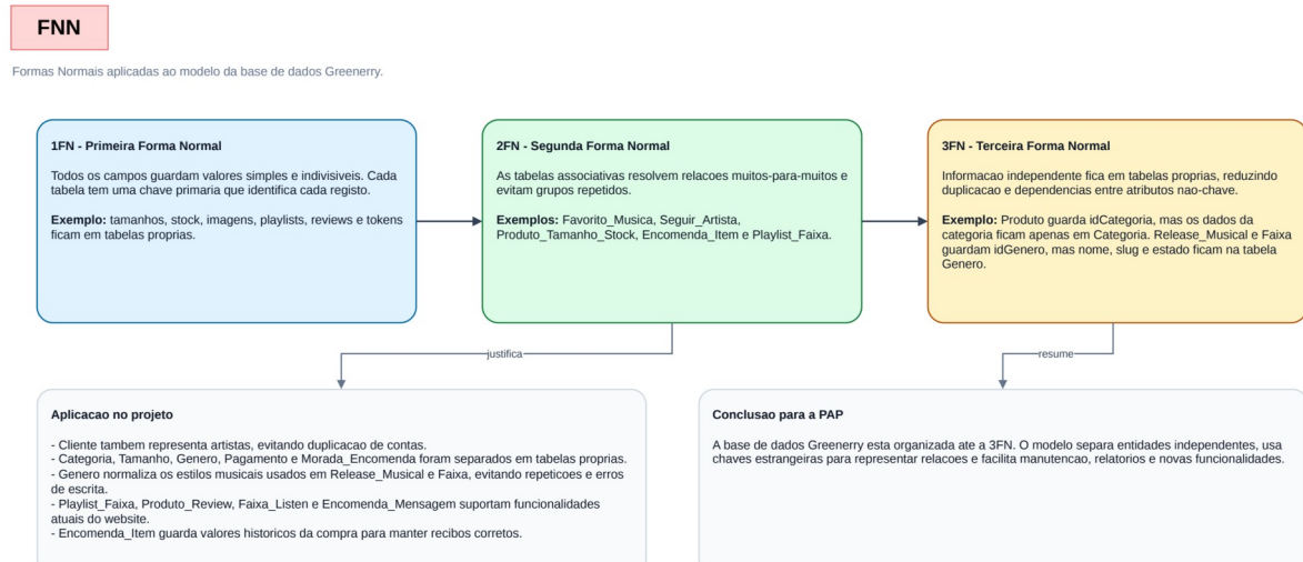
Figura 4 - Formas Normais aplicadas ao modelo da base de dados Greenerry.
