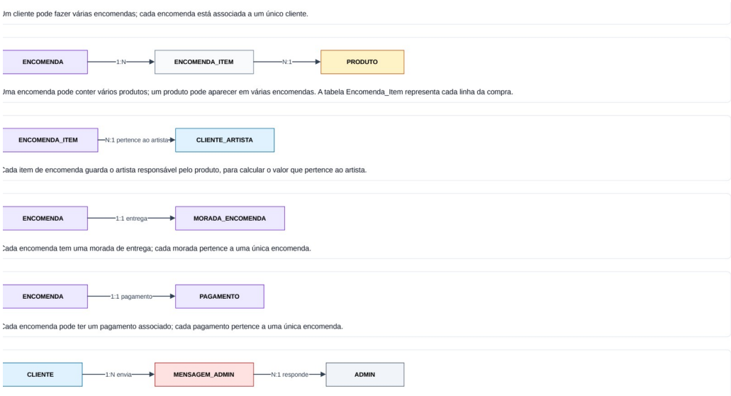
Figura 2.3 - MER detalhado, bloco 3.
