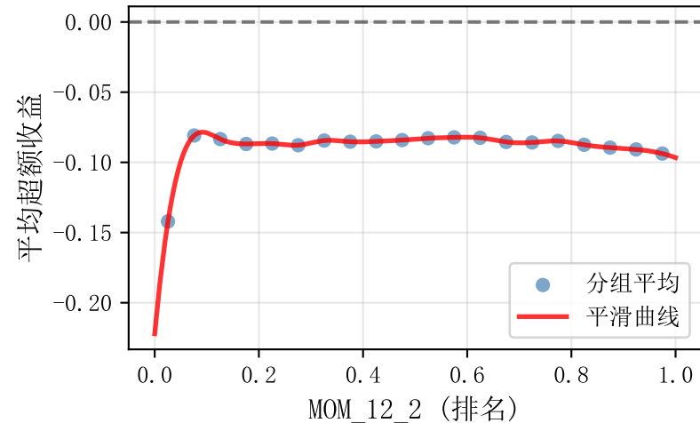
无条件关系：MOM_12_2 vs 超额收益
