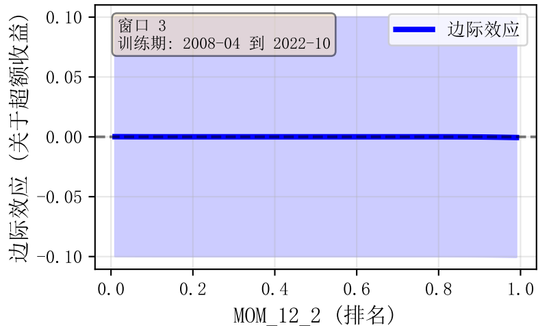
条件关系：MOM_12_2 (控制其他特征)
