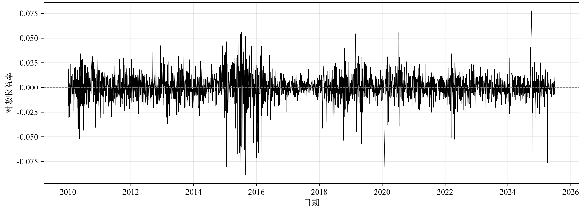
图1：上证综指对数收益率时间序列 (2010.01 – 2025.06)
