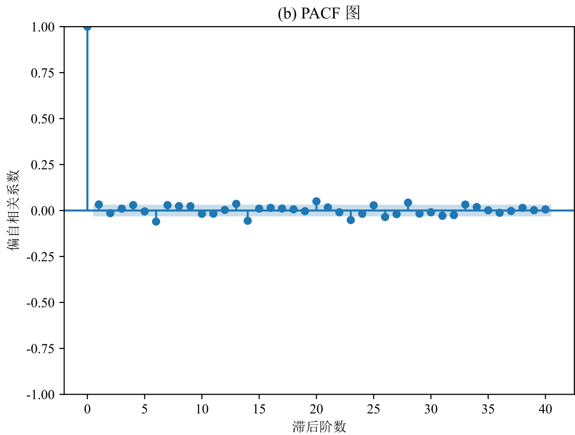
图2：对数收益率 ACF / PACF 图
