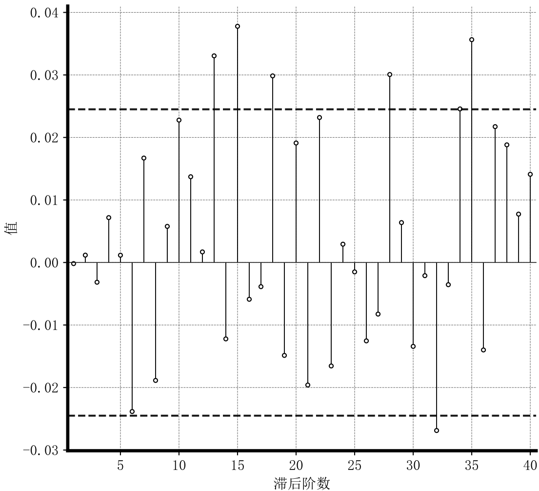
ARIMA残差 ACF
