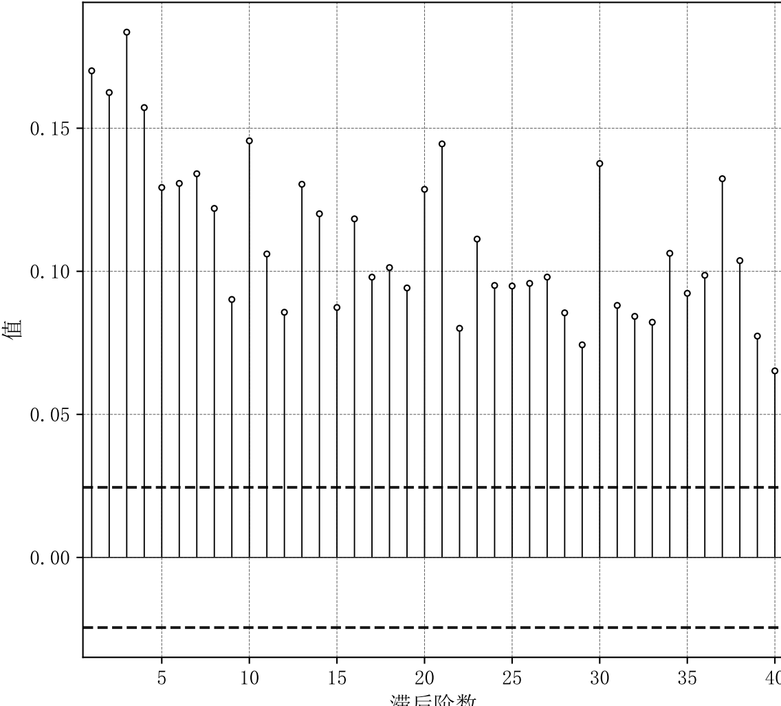
ARIMA残差 2 ACF
