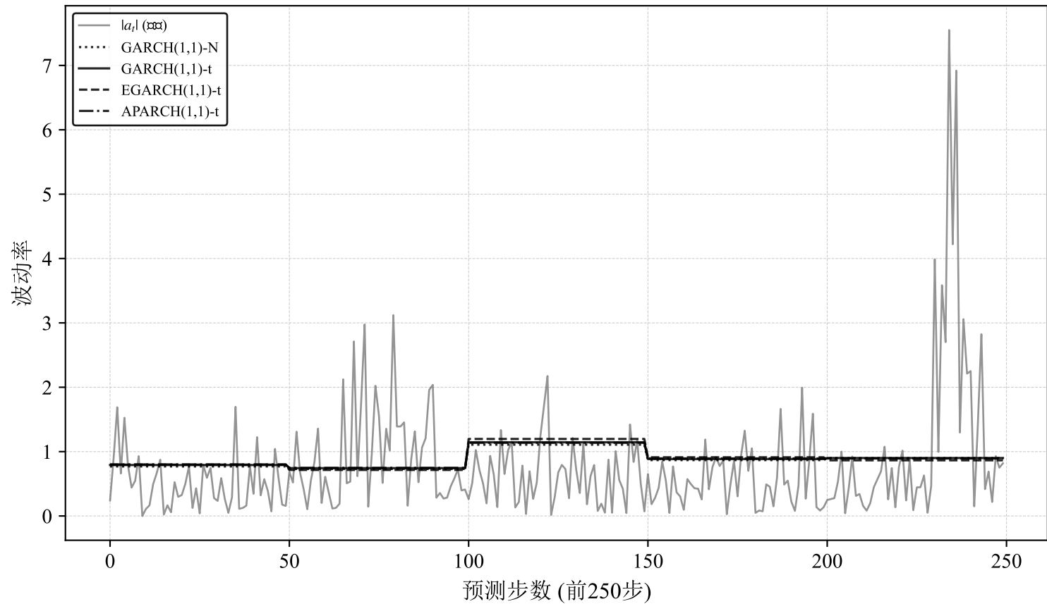
滚动窗口样本外波动率预测对比
