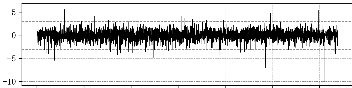
GARCH(1, 1)-t 标准化残差 ( \bar{\varepsilon}=-0.006 , \hat{\sigma}=0.992 )
