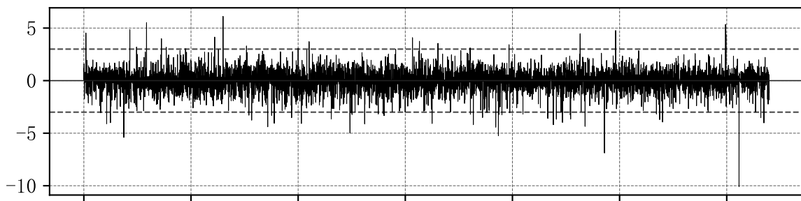
GARCH(1, 1)-N 标准化残差 ( \bar{\varepsilon}=-0.007 , \hat{\sigma}=1.000 )
