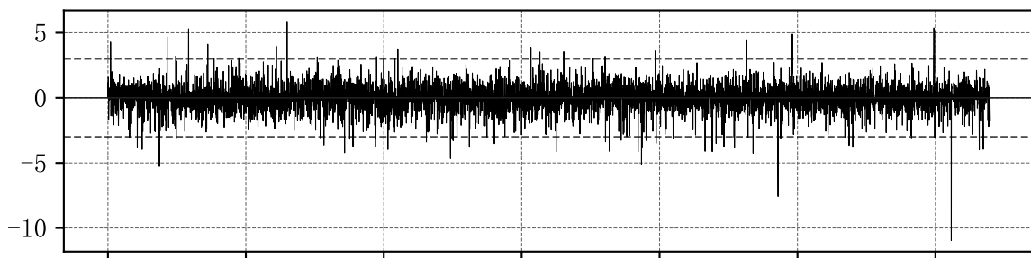
EGARCH(1, 1)-t 标准化残差 ( \bar{\varepsilon}=-0.006 , \hat{\sigma}=0.995 )
