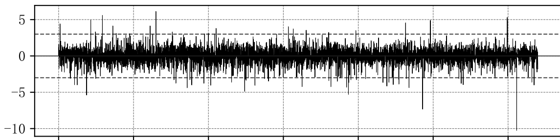
APARCH(1, 1)-t 标准化残差 ( \bar{\varepsilon}=-0.006 , \hat{\sigma}=1.010 )
