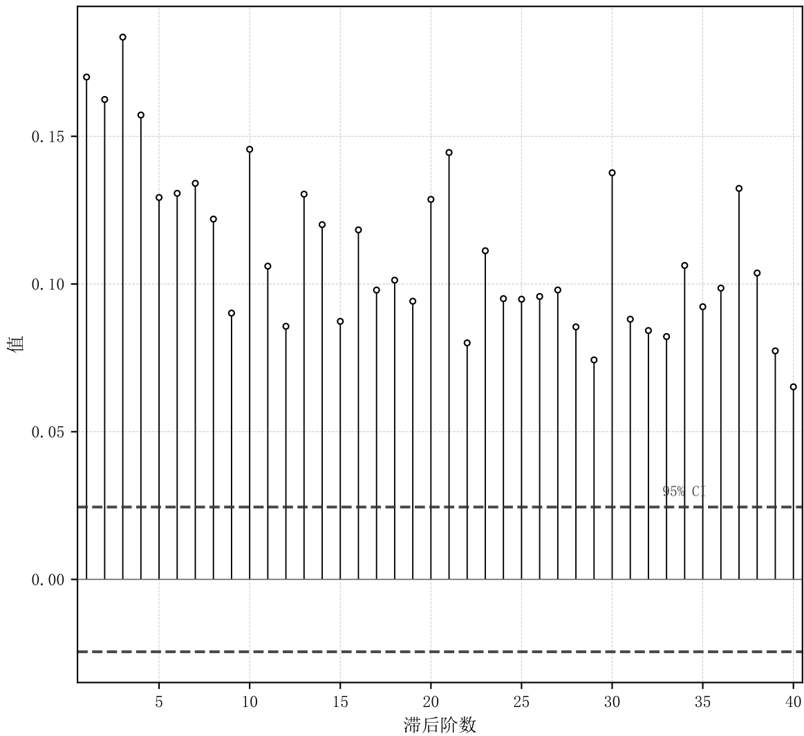
ARIMA残差 2 ACF
