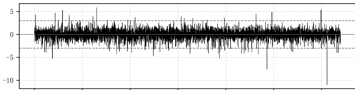
EGARCH(1, 1)-t 标准化残差 ( \bar{z}=-0.006 , \hat{\sigma}=0.995 )
