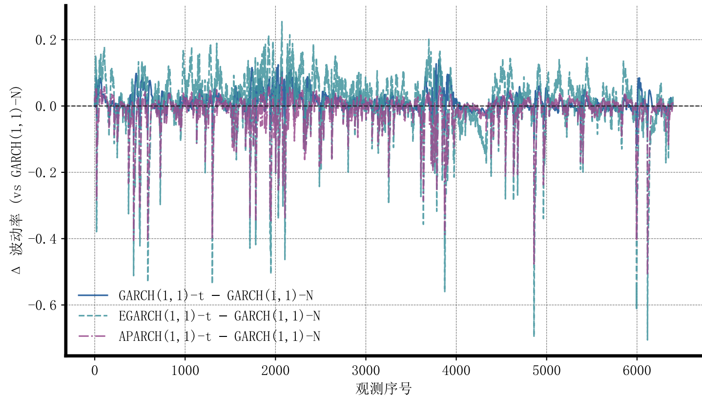
各模型与 GARCH(1,1)-N 的条件波动率差异
