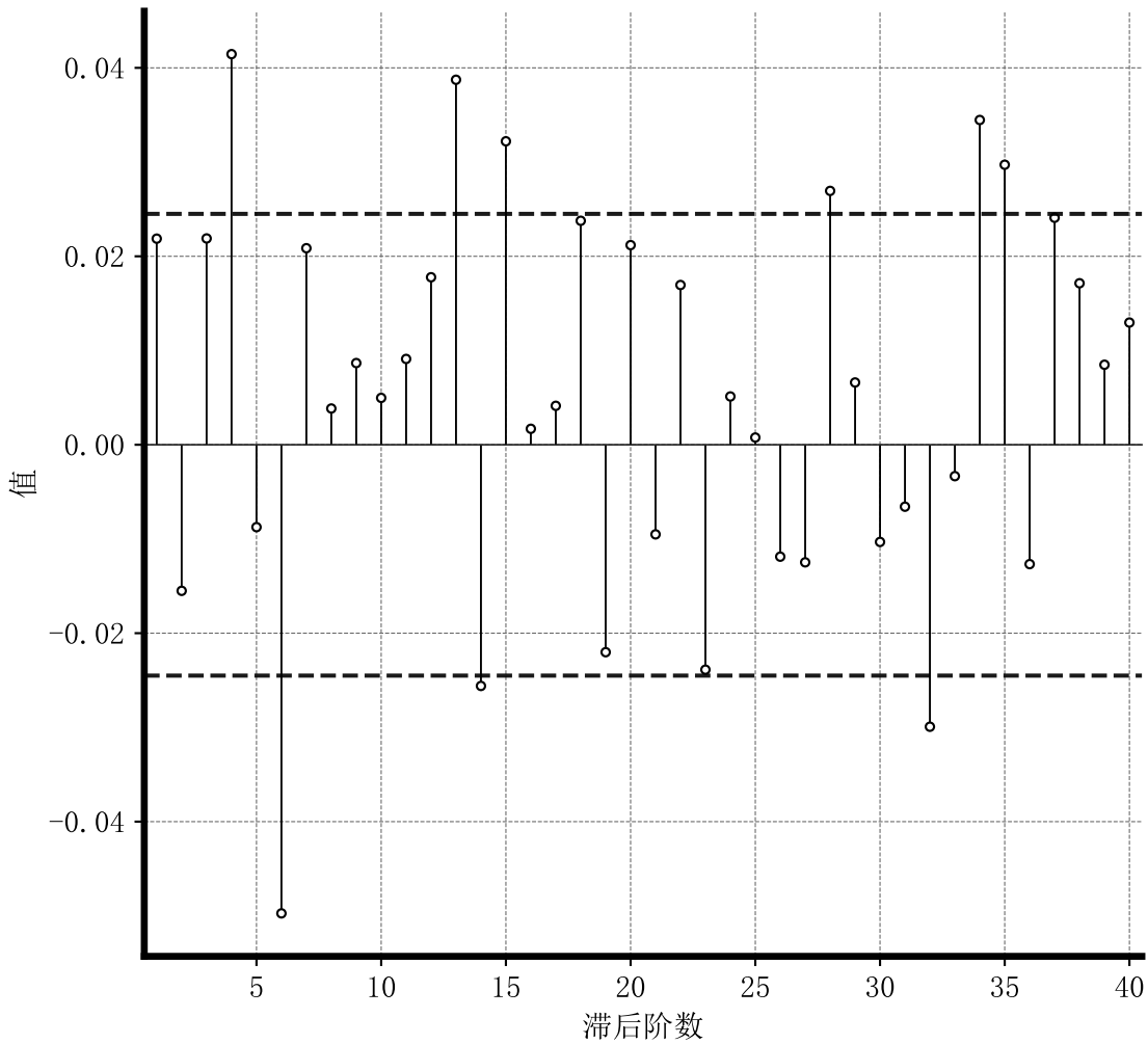
最优差分序列 PACF
