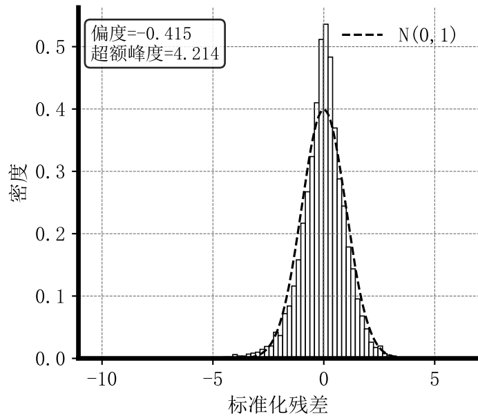
APARCH(1, 1)-t
