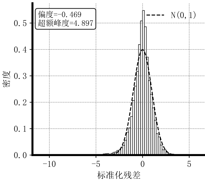
EGARCH(1, 1)-t
