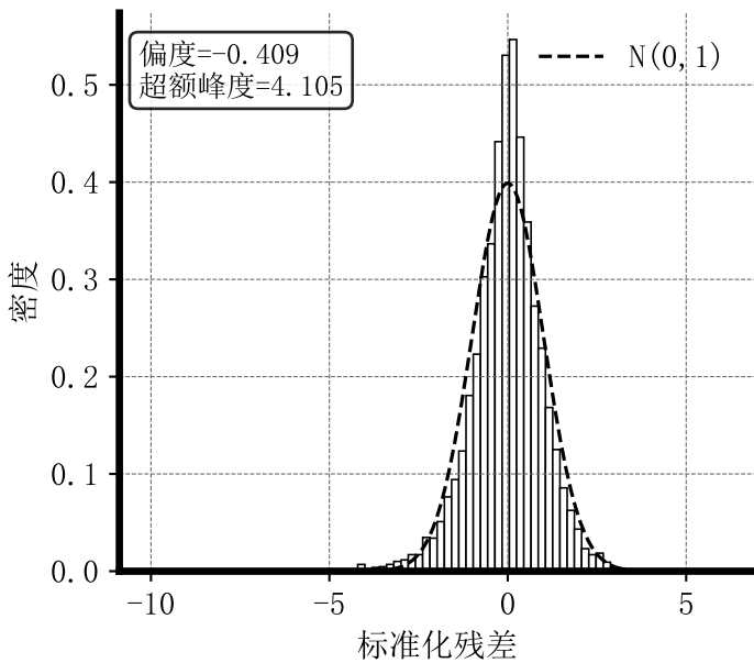
GARCH(1, 1)-N
