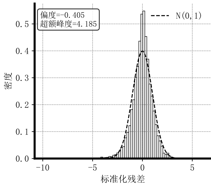
GARCH(1, 1)-t
