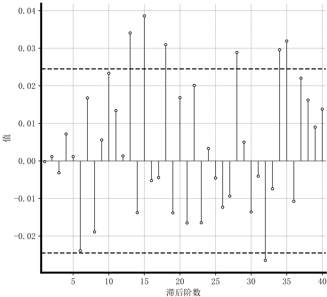
ARIMA残差 PACF
