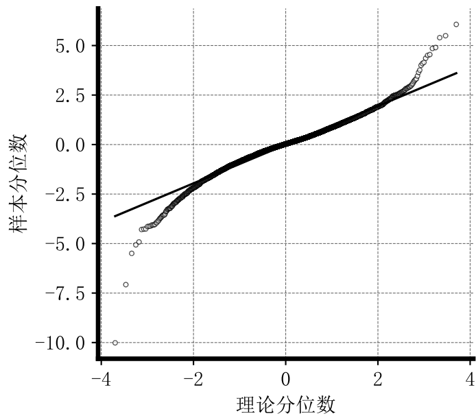
GARCH(1, 1)-t
