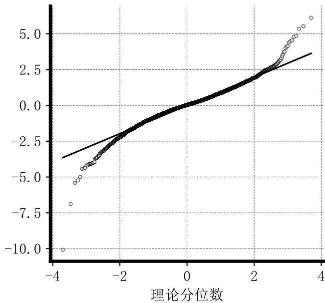
GARCH(1, 1)-N
