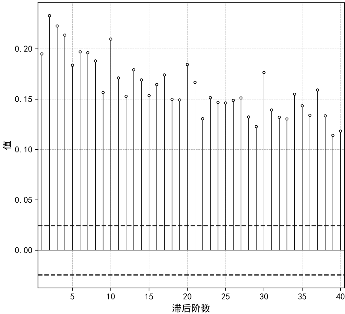
|ARIMA残差| ACF (波动聚集)
