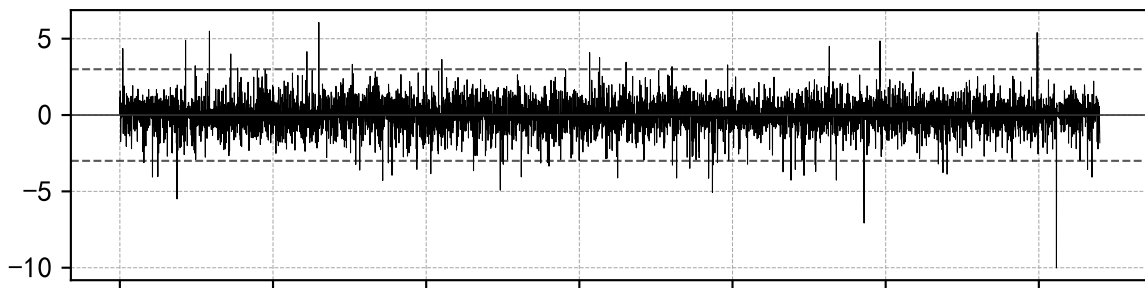
GARCH(1, 1)-t 标准化残差 ( \bar{\mu}=-0.006 , \hat{\sigma}=0.992 )
