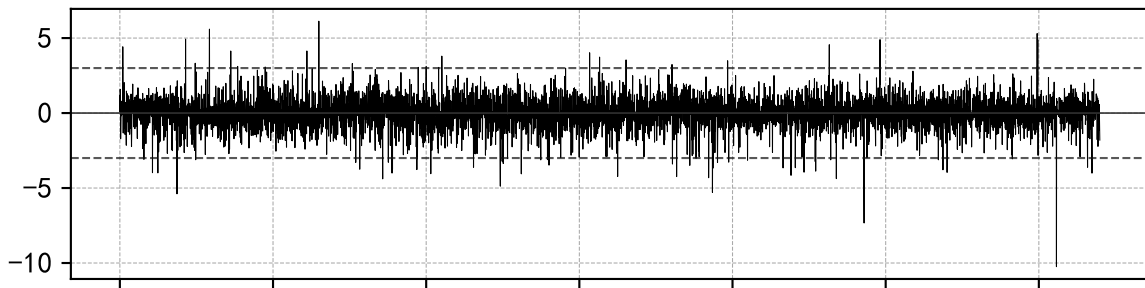
APARCH(1, 1)-t 标准化残差 ( \bar{\mu}=-0.006 , \hat{\sigma}=1.010 )
