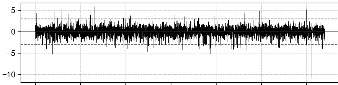
EGARCH(1, 1)-t 标准化残差 ( \bar{\mu}=-0.006 , \hat{\sigma}=0.995 )
