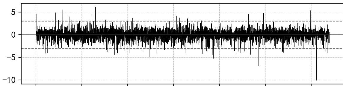
GARCH(1, 1)-N 标准化残差 ( \bar{\mu}=-0.007 , \hat{\sigma}=1.000 )
