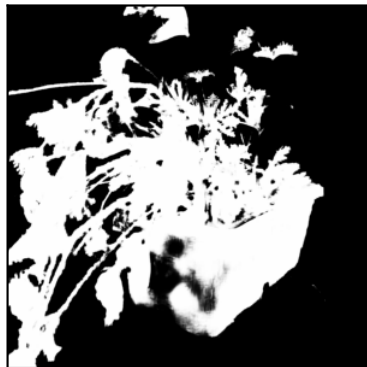
SMat-auto
