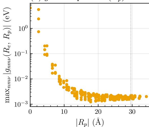
(d) g : côté phonon ( R_p )
