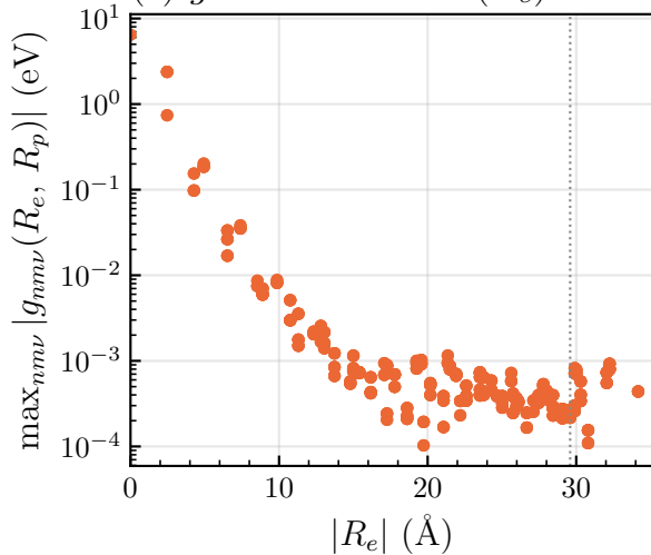
(c) g : côté électron ( R_e )
