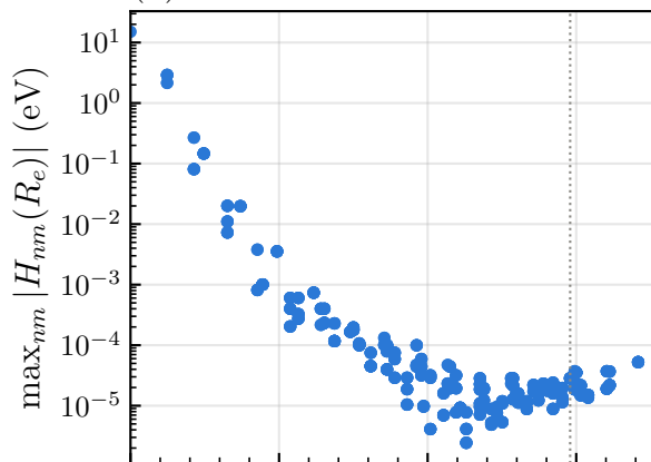
(a) H : hamiltonien
