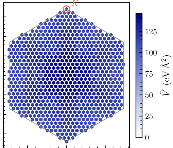
(d) \pi : M^{NL} le long de M
