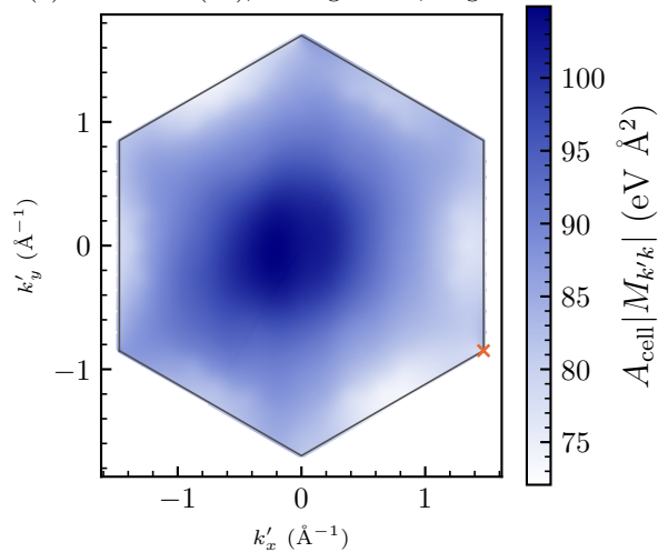
(d) conduction ( \pi^* ), Kumagai-Oba, Wigner-Seitz
