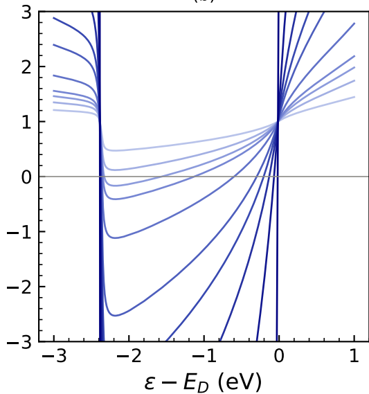
(b) \text{Re } \lambda (valeur propre non triviale)
