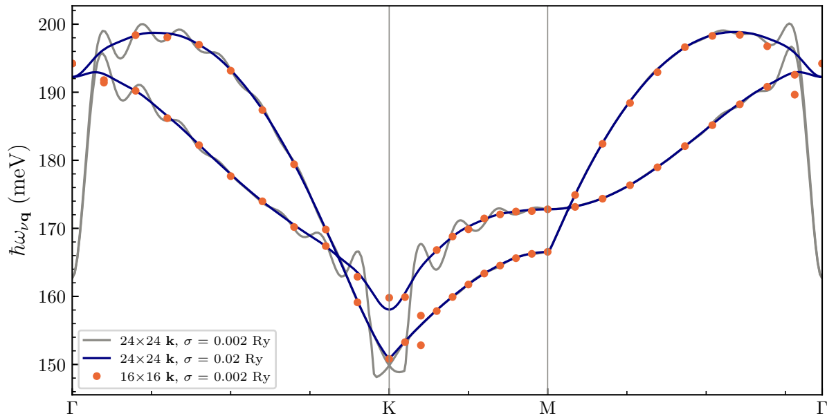
Anomalies de Kohn en fonction de l'élargissement de Marzari-Vanderbilt \sigma
