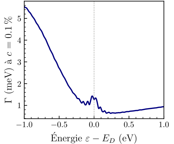
(f) Lacune, c = 0.1\% (vs Kaasbjerg ordre de grandeur seulement)
