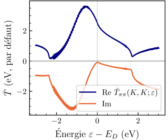
(d) \bar{T} en K , paire \pi (trace/2)
